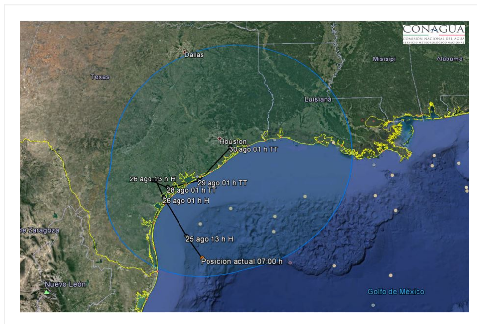
Traectoria pronóstico del Huracán cat. 2 "Harvey"
